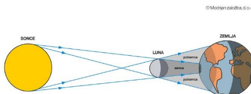
Položaj Sonca, Lune in Zemlje ob Sončnem mrku
